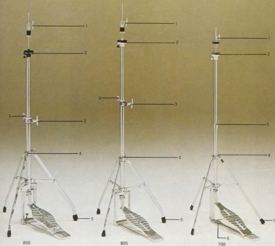
■800ハイハットスタンド .....¥10,000
