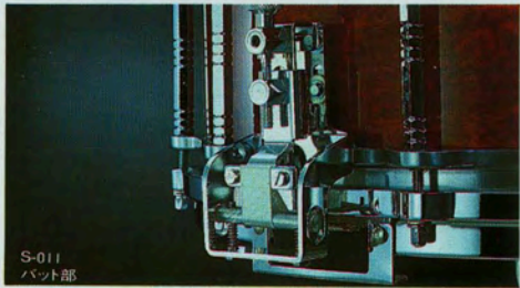
S-011 ストレイナー部
