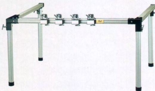
DR-1 : 700mm/ 27"(H)X1360mm/53"(W)X1200mm/46½"(D)
