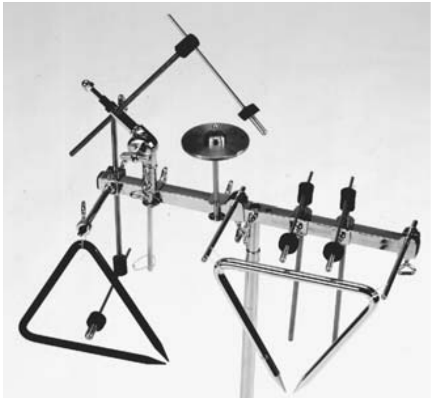
Diverse Anschlagmöglichkeiten für Triangeln mit Hilfe der Anschlagvorrichtung Nr. 249 (incl. Nr. 248) sowie für Crotales (siehe S. 89) Nr. 249 C mit Schrägsteller Nr. 253
