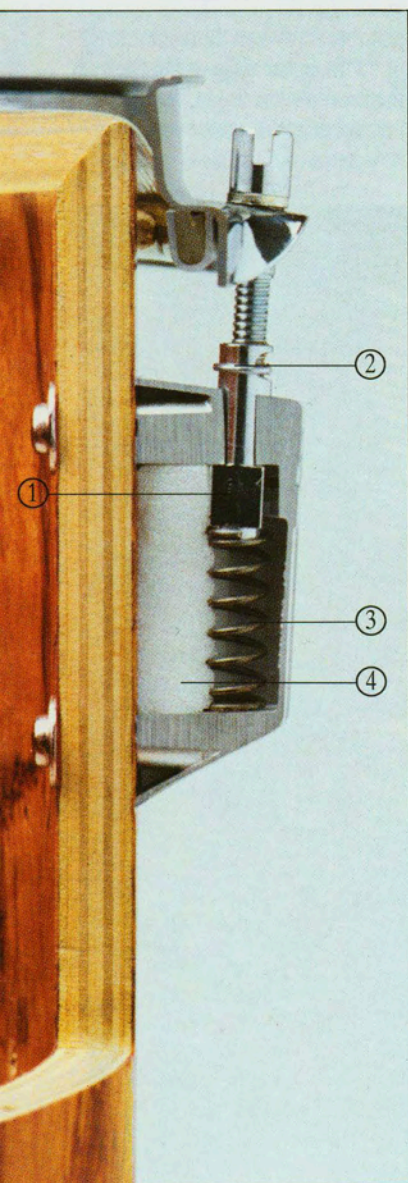
Cutaway of a Sonor lug
